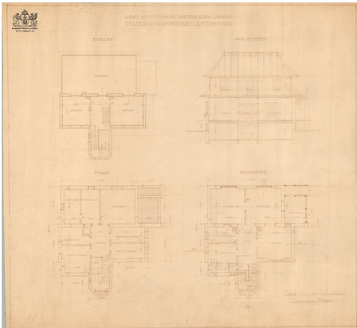
A váci Kertvárosba tervezett „hatszobás” mintaház szintenkénti alaprajzai és metszete. HU BFL XV.17.f.336.a – 21, 1-10. főlő
