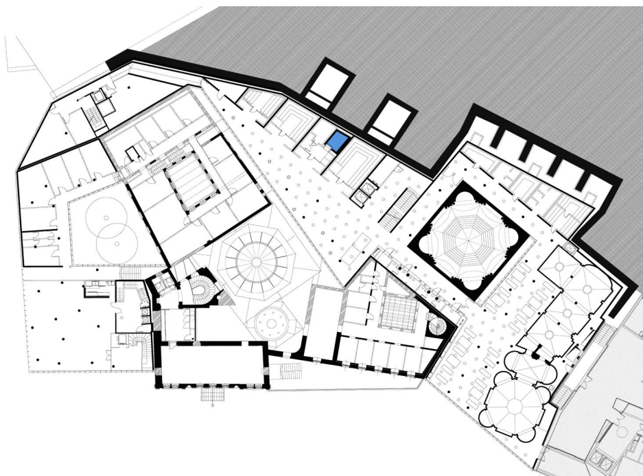
Pincésinti alaprajz
