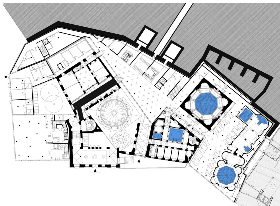
Földszinti alaprajz
