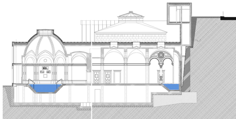
Hosszmetszet a Zuhanycsarnokon át
