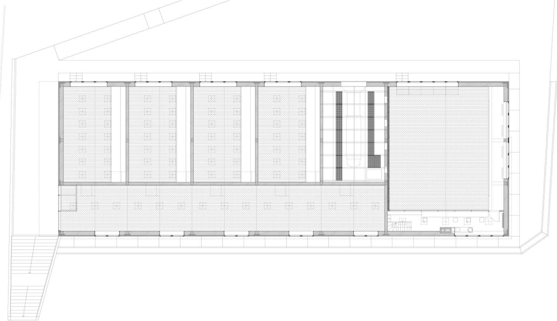
Galériaszint alaprajza
