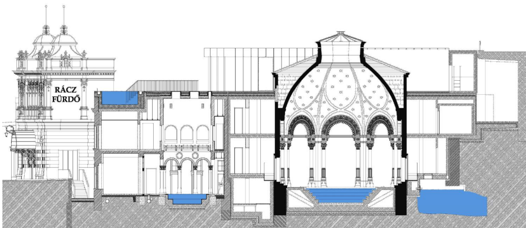
Keresztmetszet a Flórafürdőn és az Ybl melegvizes csarnokon át
