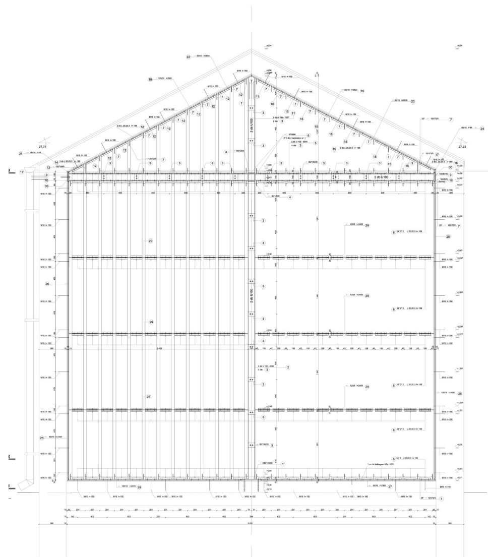
Fix portál terve
