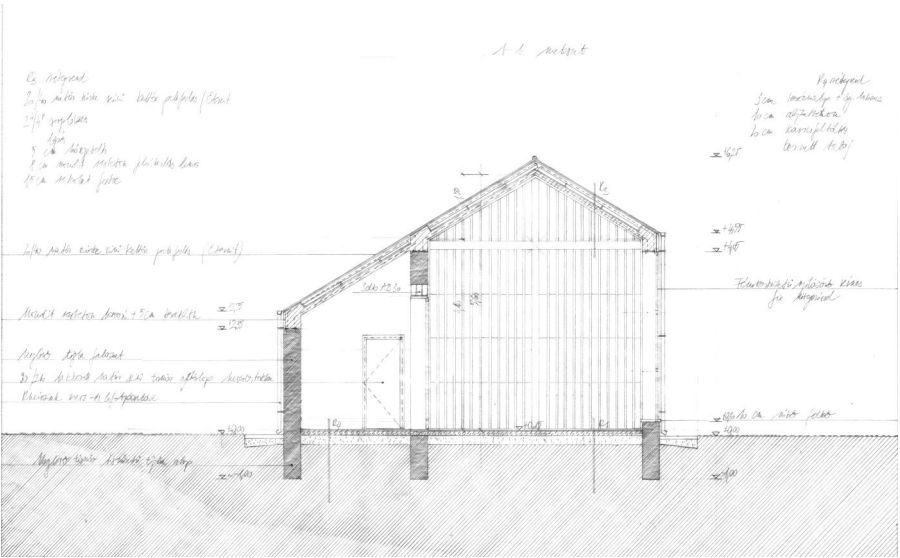
Keresztmetszet
