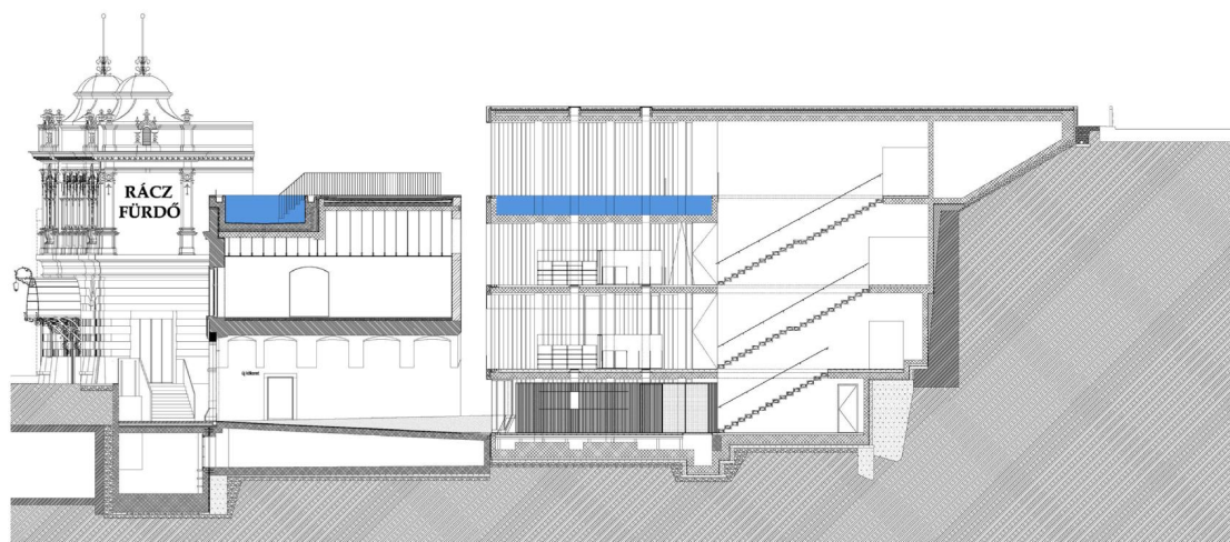
Keresztmetszet a Barokk Kapualjón és a Szitán át
